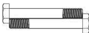
(20) Шестигранный болт: М10×72 — 2 шт.
