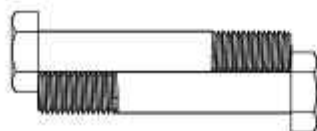
(23) Шестигранный болт: М10×52 — 2 шт.
