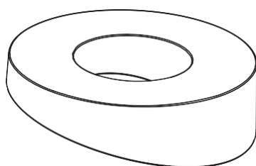
Одна шайба Φ23.5*Φ10.5*7.1 (#16)
