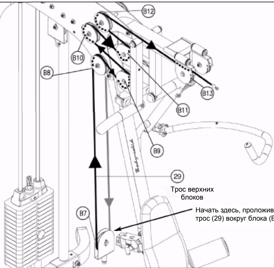
Диаграмма 1 Установка троса
